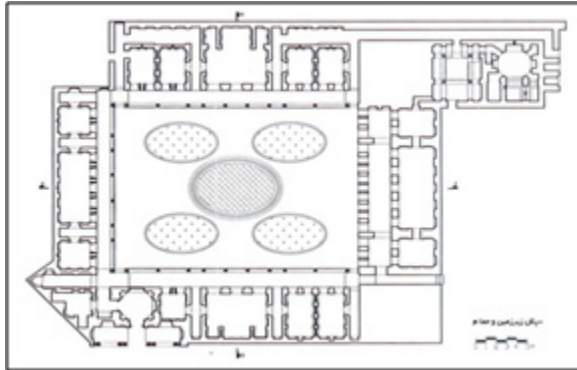
پلان ۱: حیاط بیرونی (قلعه خدارحم خان) چالستر (فتح‌اللهی، ۱۳۸۸: ۸۶-۸۷).
